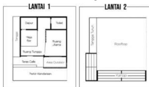
Gambar 3. Desain Denah Terpilih Lantai 1 dan 2
