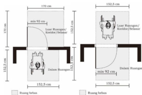
Gambar 1. Lebar Efektif Pintu Serta Ruang Bebas
