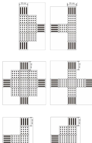
Gambar 11. Contoh Ukuran dan Jenis Jalur Pemandu
