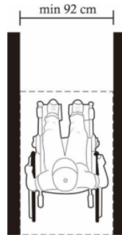
Gambar 5. Lebar Efektif Koridor
