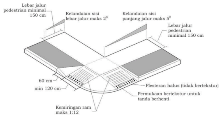
Gambar 8. Dimensi Ram Pada Jalur Pedestrian
