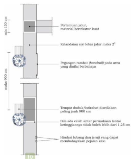
Gambar 6. Prinsip Perencanaan Jalur Pedestrian
