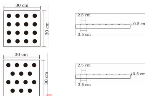
Gambar 9. Tipe Tekstur Ubin Peringatan
