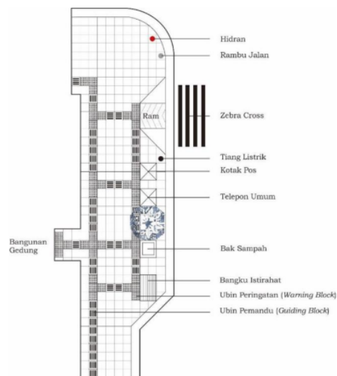
Gambar 12. Prinsip Perencanaan Jalur Pemandu
