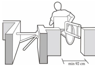
1 Gambar 2. Lebar Efektif Pintu Akses
