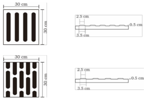
Gambar 10. Tipe Tekstur Ubin Pengarah
