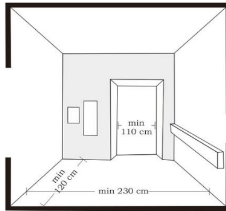
Gambar 17. Detail Lift Dalam Lift Penumpang
