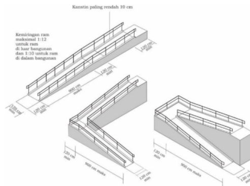
Gambar 15. Varian Bentuk Ram
