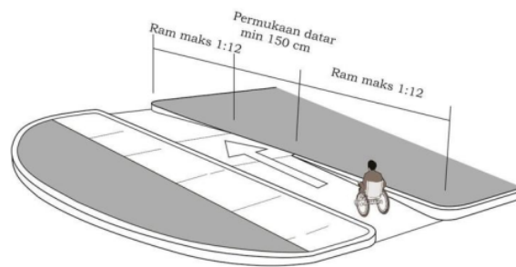
Gambar 7. Sudut Kemiringan Maksimal Ram Pada Jalur Pedestrian
