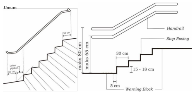
Gambar 14. Detail Tangga Yang Direkomendasi
