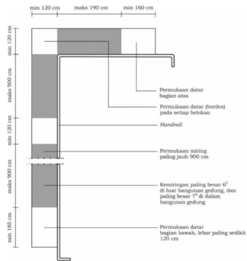
Gambar 16. Persyaratan Ram
