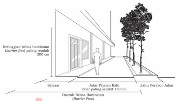
1 Gambar 4. Contoh Selasar dengan Satu Dinding Pembatas
